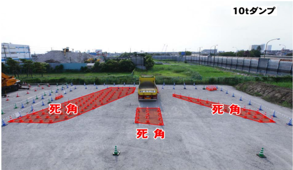
10 tダンプの死角の見える化
