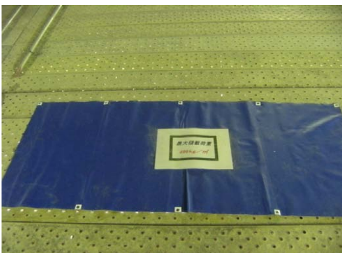
材料置き場シートの積載荷重表示 ハト目で枠組み足場上部に結束
