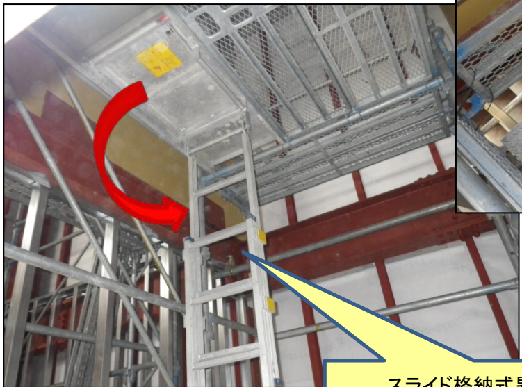
スライド格納式昇降タラップ
