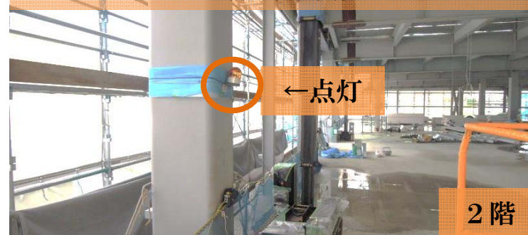
通行路上部死角設置ランプ
