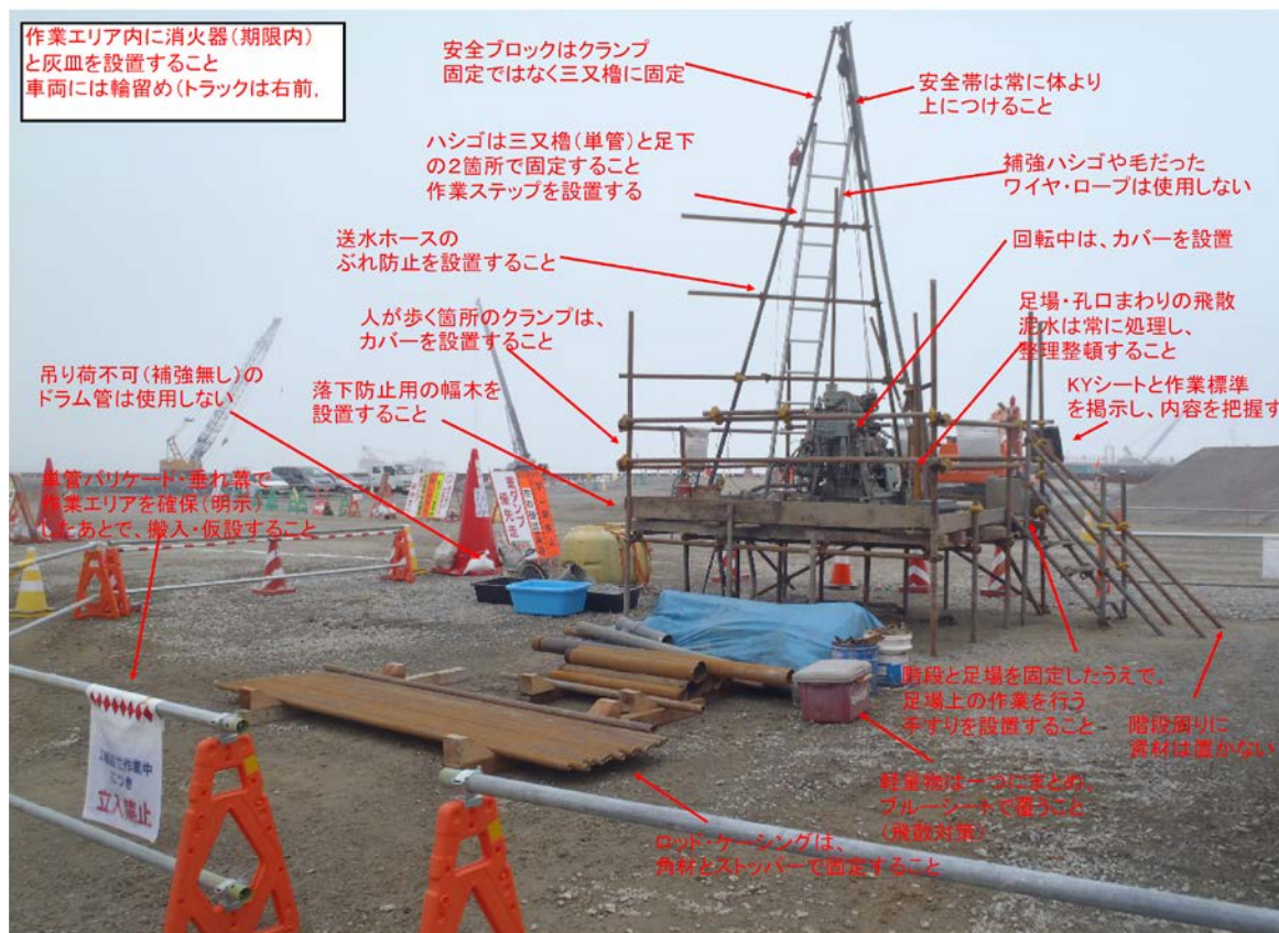
写真-2 安全なボーリング足場の説明図
