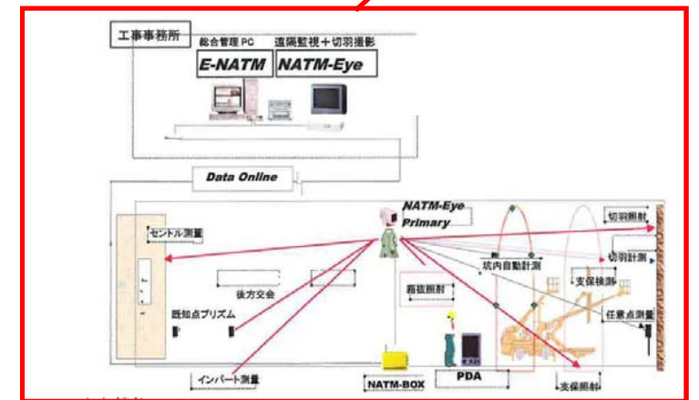
現場計測システム概要
