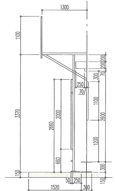
断面 s=1/40
