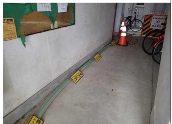
仮設給水ホース配置・注意喚起看板
