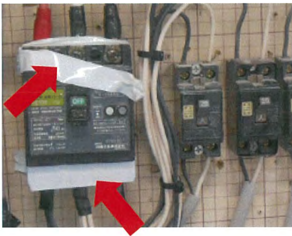
紛失した端子カバーをビニルテープで補修
