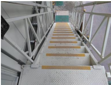
現場事務所階段の防滑対策標準化(2) 六丁の目建築作業所
