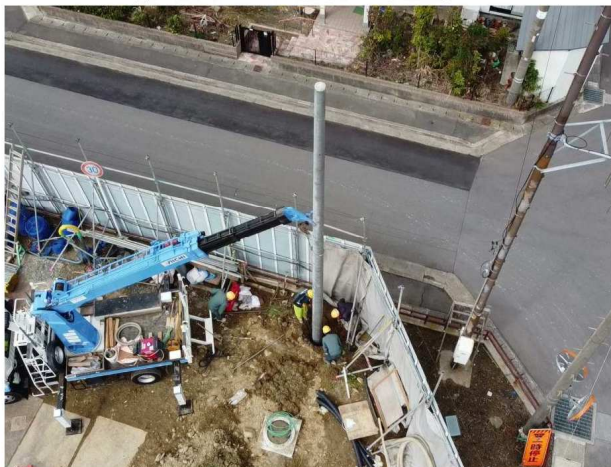
【建柱 状況】
