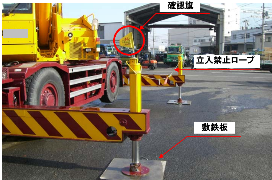
アウトリガー 張出し状況
