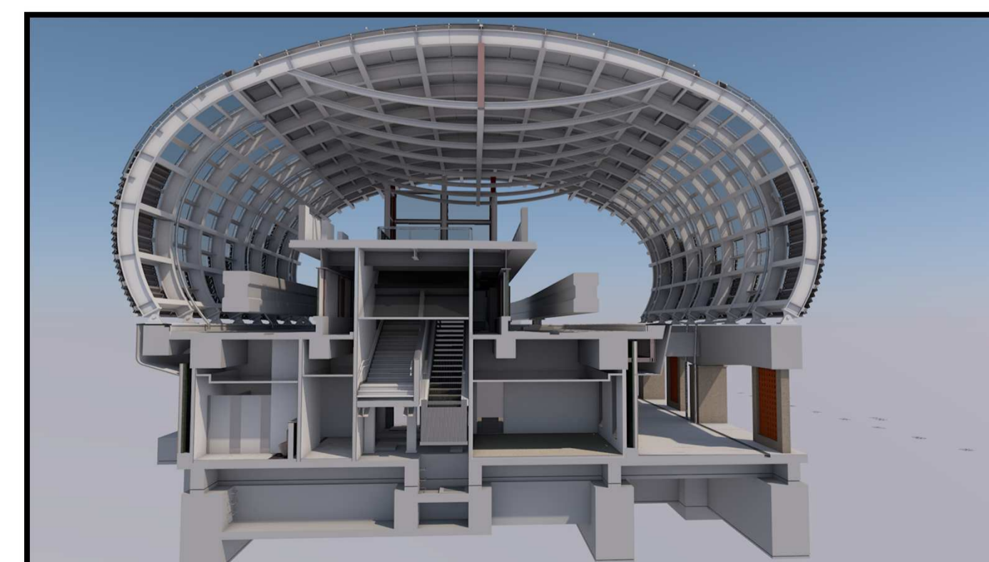
図.3 断面パース
