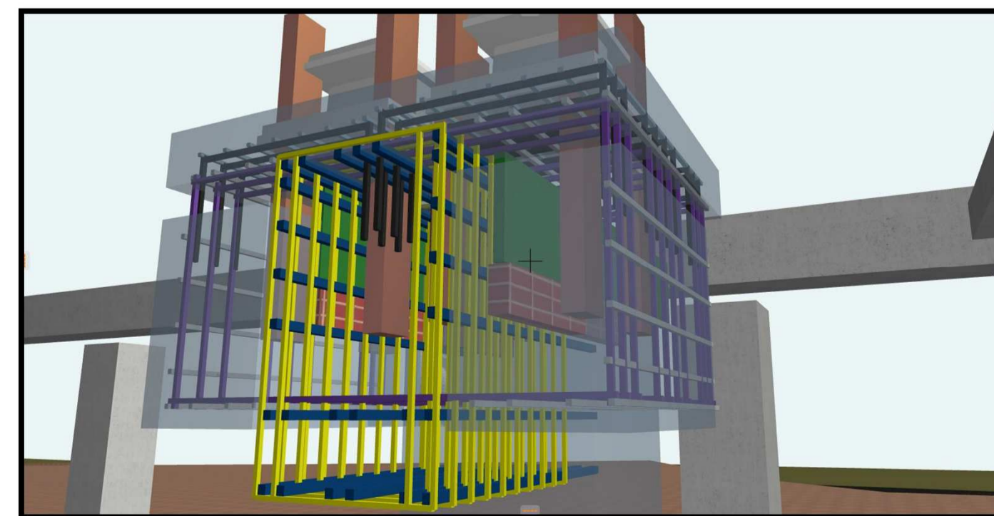
図.2 支承内部鉄筋収まり検討パース
