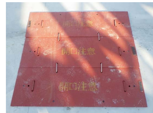
建屋内の鉄板蓋による養生
