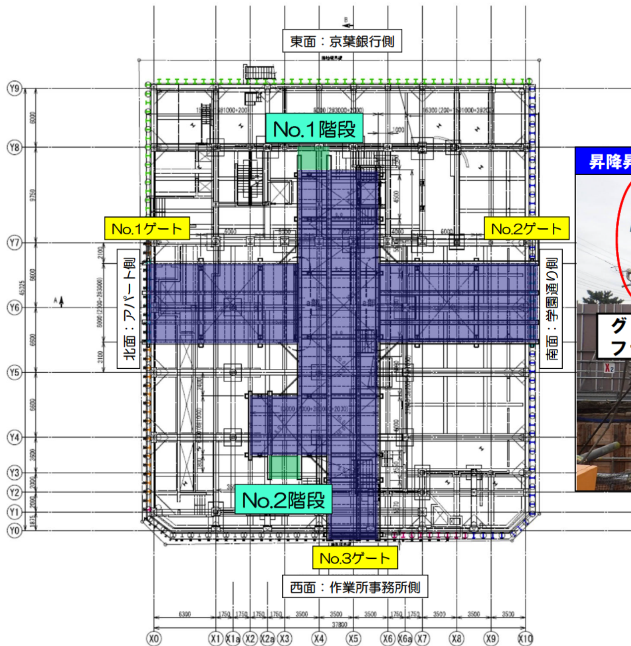
乗入構台・昇降設備計画
