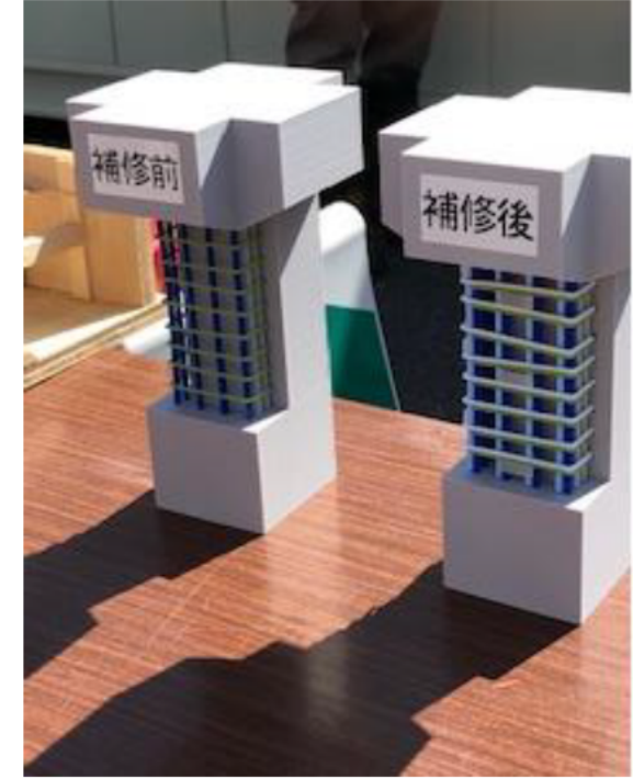
3Dプリンターによる補修前後の模型
